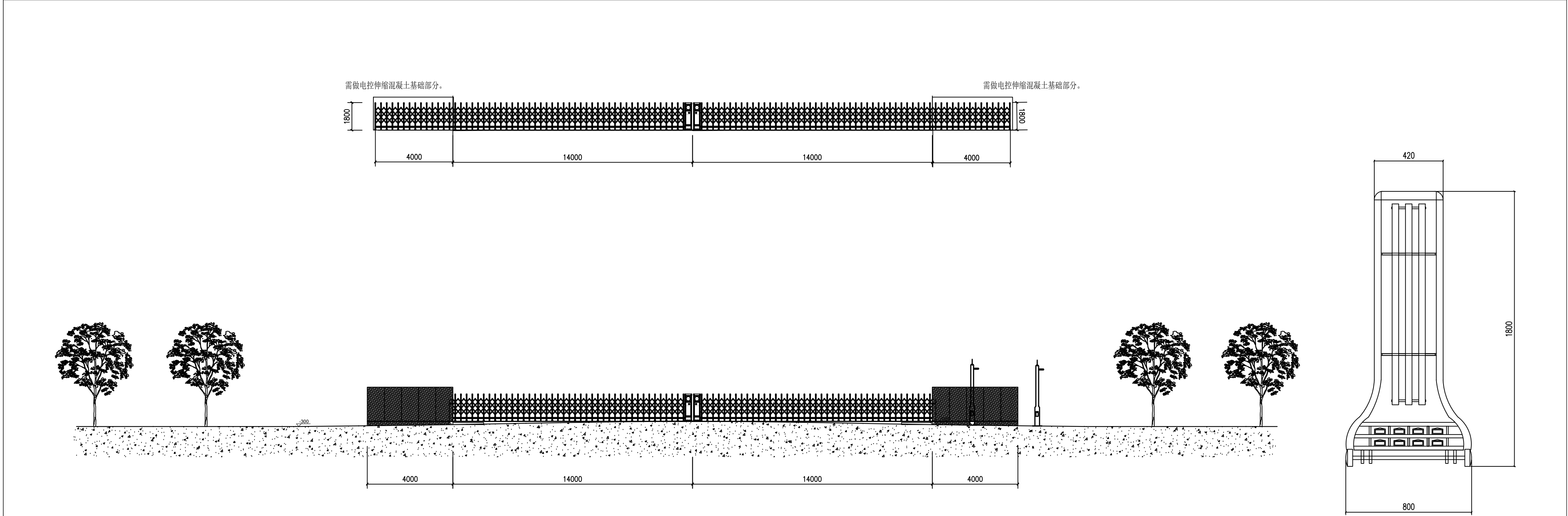
立面安装示意图
